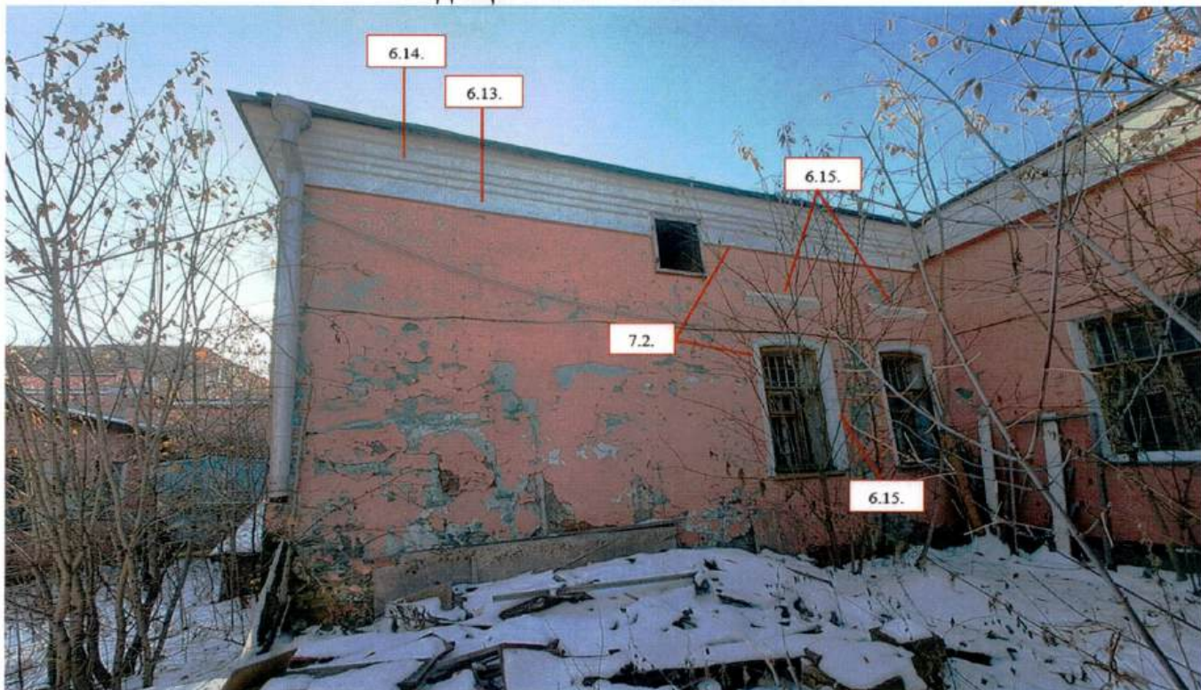
Северный фасад основного объема «Бывший жилой дом» объекта «Жилой дом», входящего в состав ансамбля
